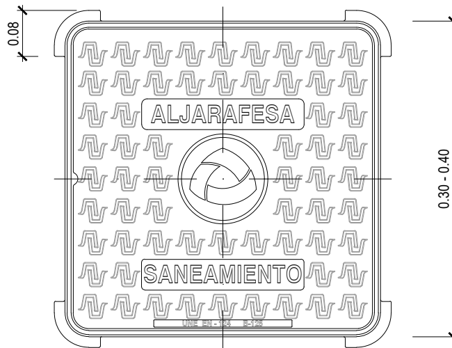
PLANTA TAPA
