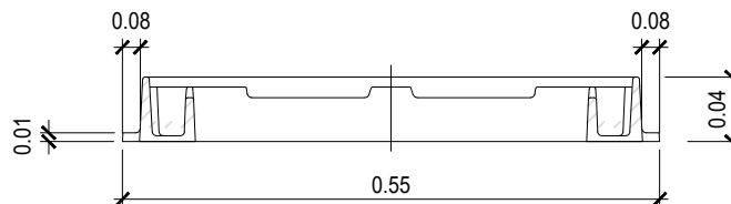
SECCIÓN MARCO
