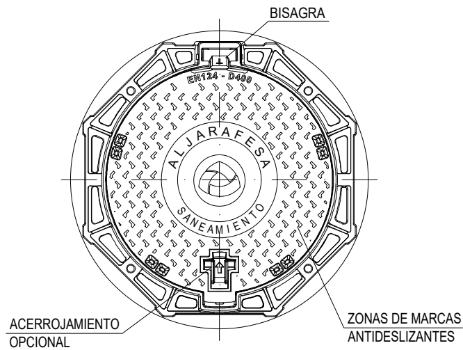
PLANTA
