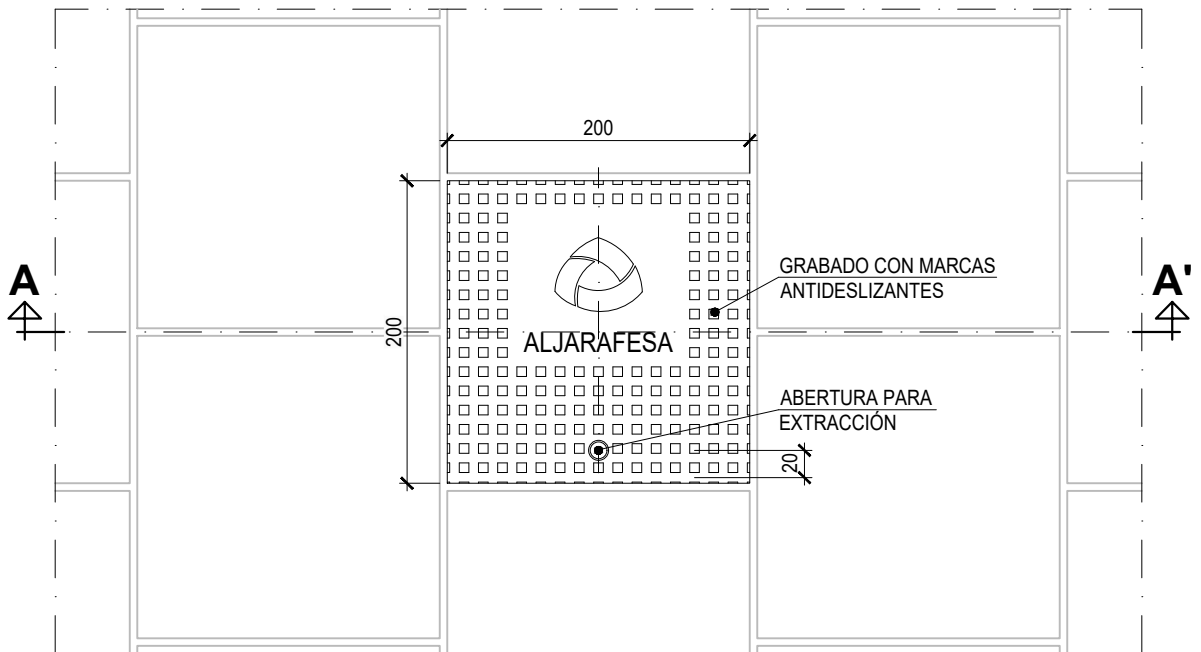
PLANTA
