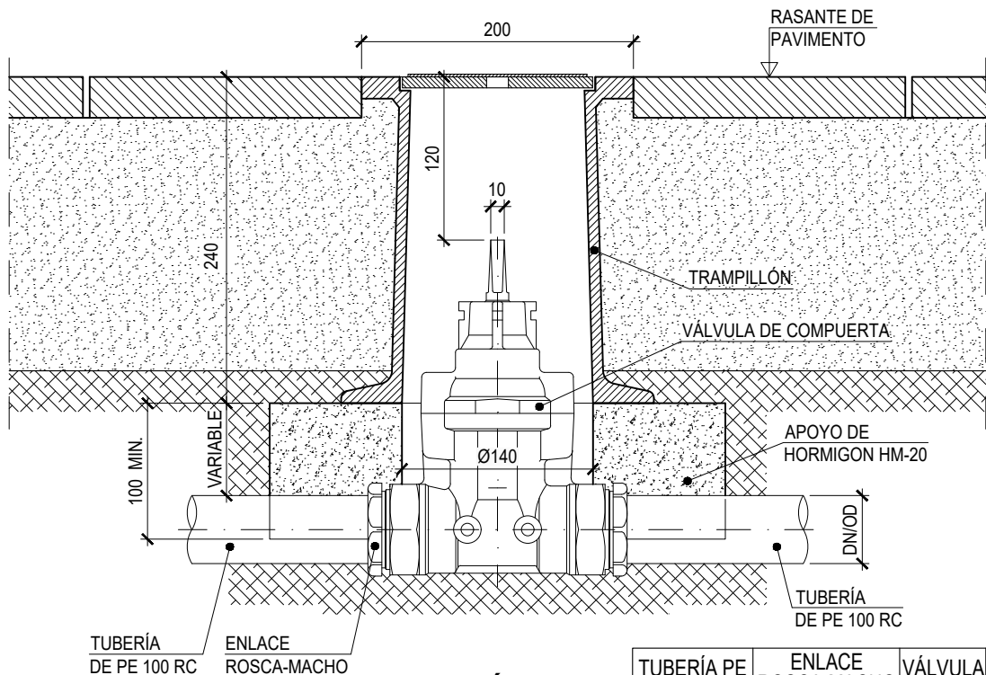
SECCIÓN A-A'
